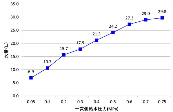
[流量測定 (二次側圧力を 0.3MPa に設定)]
