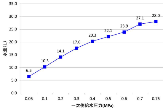
[流量測定 (二次側圧力を 0.2MPa に設定)]
